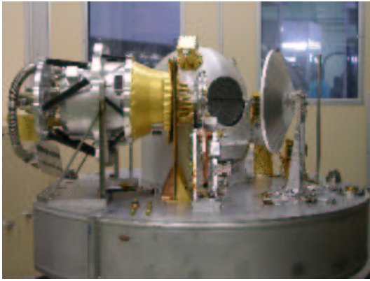
Figure 1: Instrument de qualification de PLANCK-HFI sur sa platine d'étalonnage (cf. http://planck.fr/ ).
